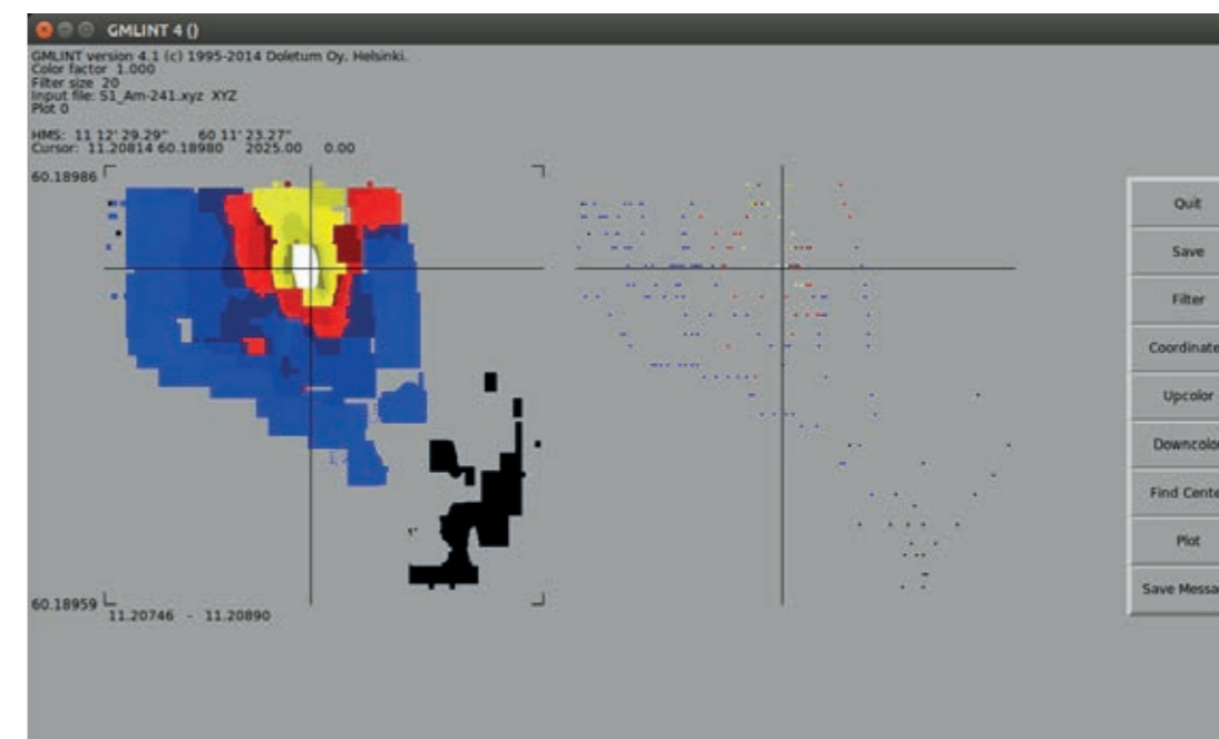
Kuva 6. Alue S1. GMLINT-ohjelmalla on mallinnettu säteilypinta (Am-241). Mittauspisteet ovat kuvassa oikealla. Kursori osoittaa aktiivisinta kohtaa, ja aktiivisuusarvo (2025) ja sen koordinaatit ovat luettavissa kuvasta.
