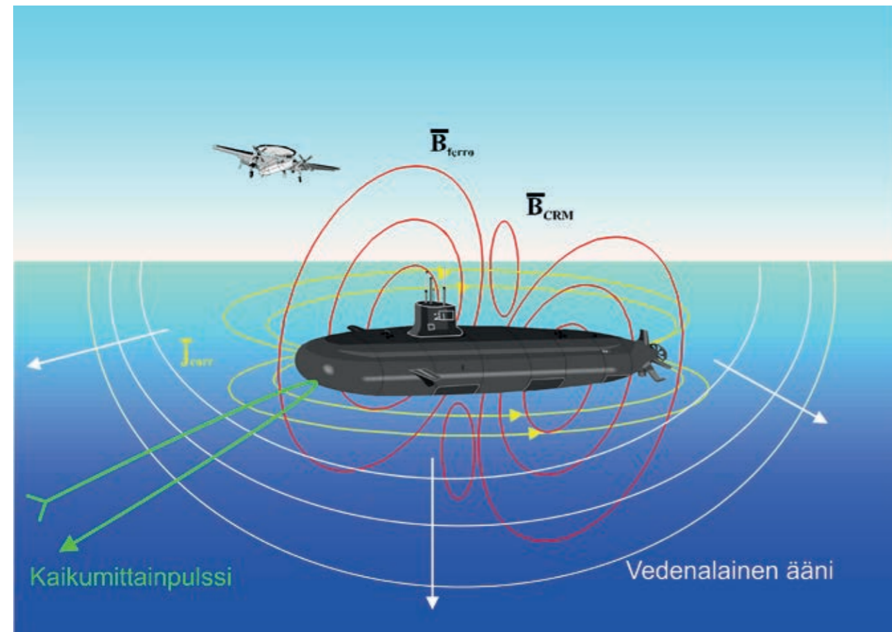
Kuva 1. Sukellusveneeseen akustiset, magneettiset ja sähköiset herätteet.
